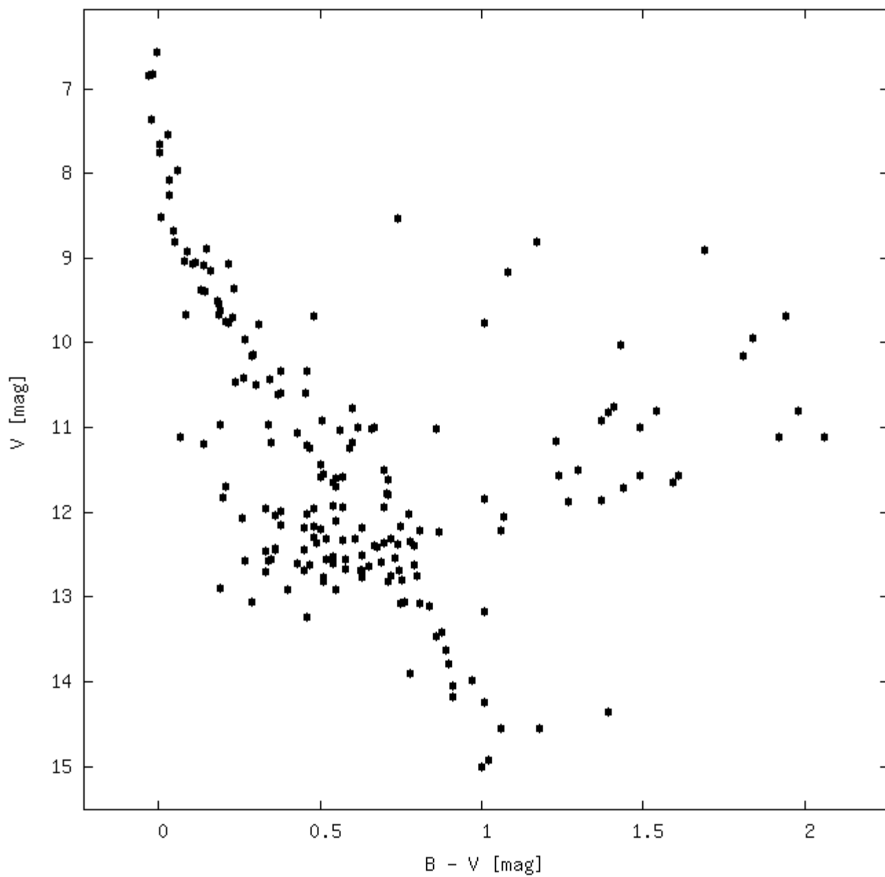
NGC 7092
