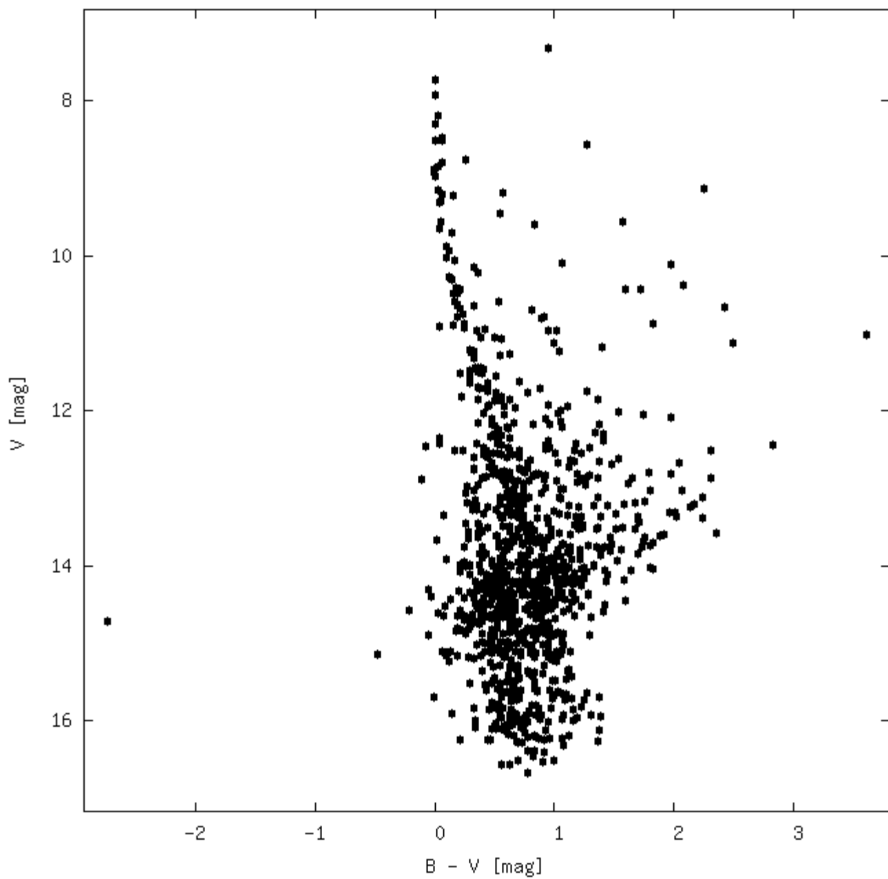
NGC 1039
