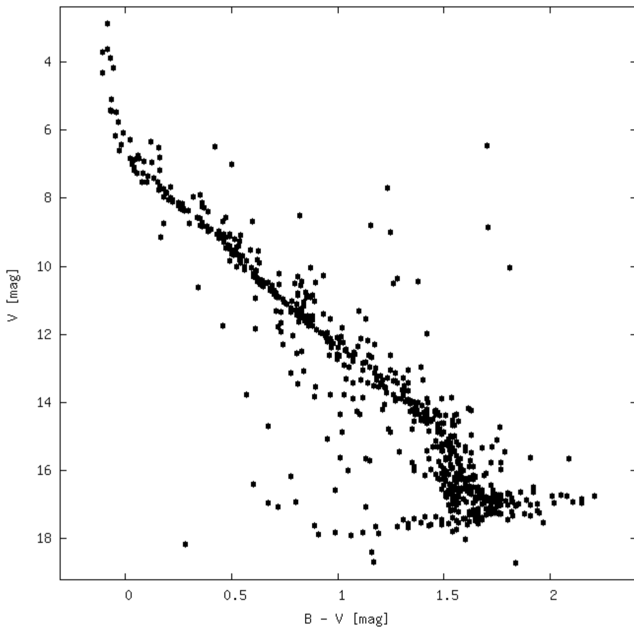
Pleiades
