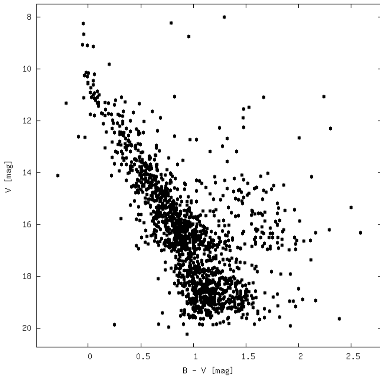
NGC 2301
